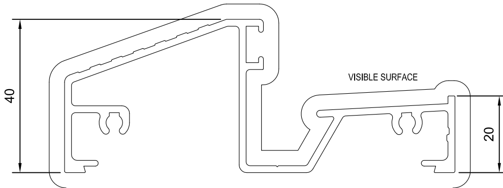
AS2370 HINGED DOOR INWARD OPENING
