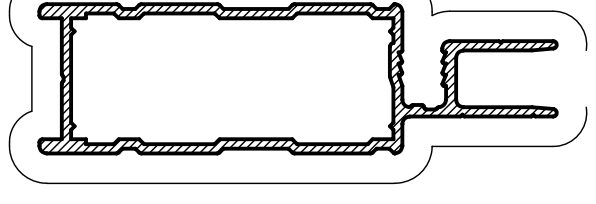
SD8 DOOR FRAME Mass. 0,629 Kg/m Anod. Per. 232 Paint Per. 197
