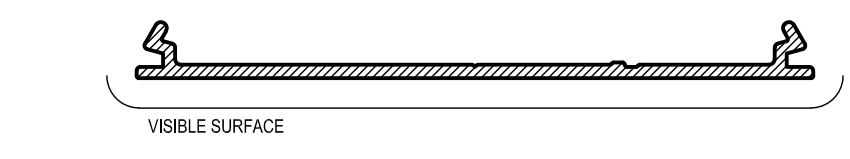
AS5 FLAT INFILL
