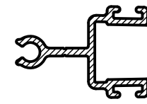
SDH017 STILE PVC 10mm x 3m
