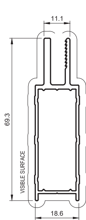
SD60 ALU-GARD EDGE DOOR FRAME Anod. Per. 228 Paint Per. 175
