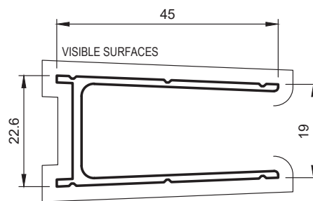
1414104 DOOR ADAPTOR
