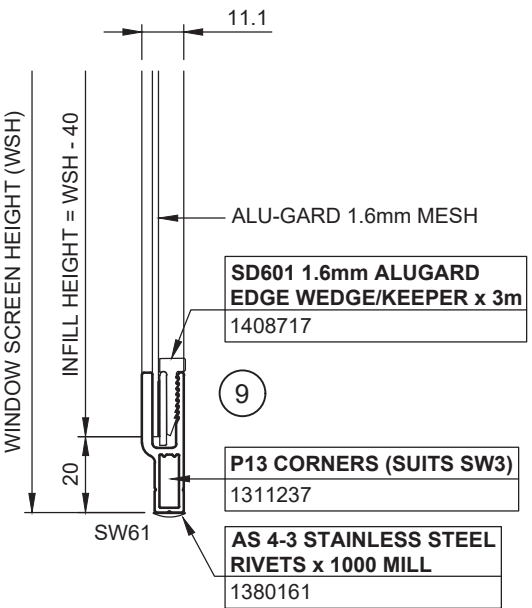
SW61 9mm FRAME
