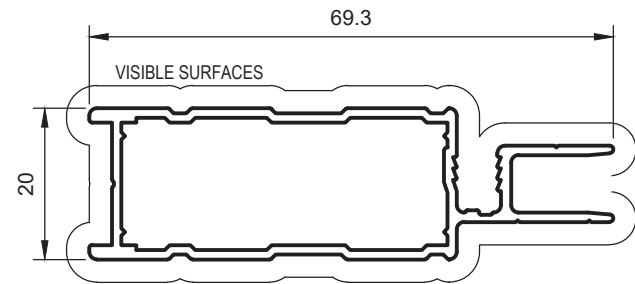
SD8 DOOR FRAME Anod. Per. 232 Paint Per. 197
