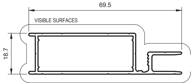
SD2 DOOR FRAME Anod. Per. 228 Paint Per. 194
