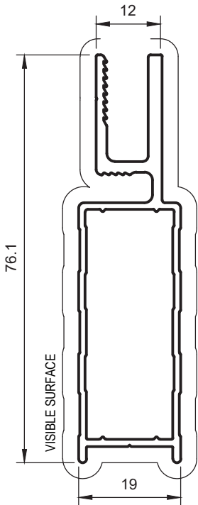
SD50 COMBO DOOR FRAME STD
