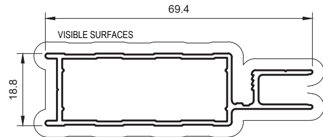
SD9 DOOR FRAME Anod. Per. 227 Paint Per. 192
